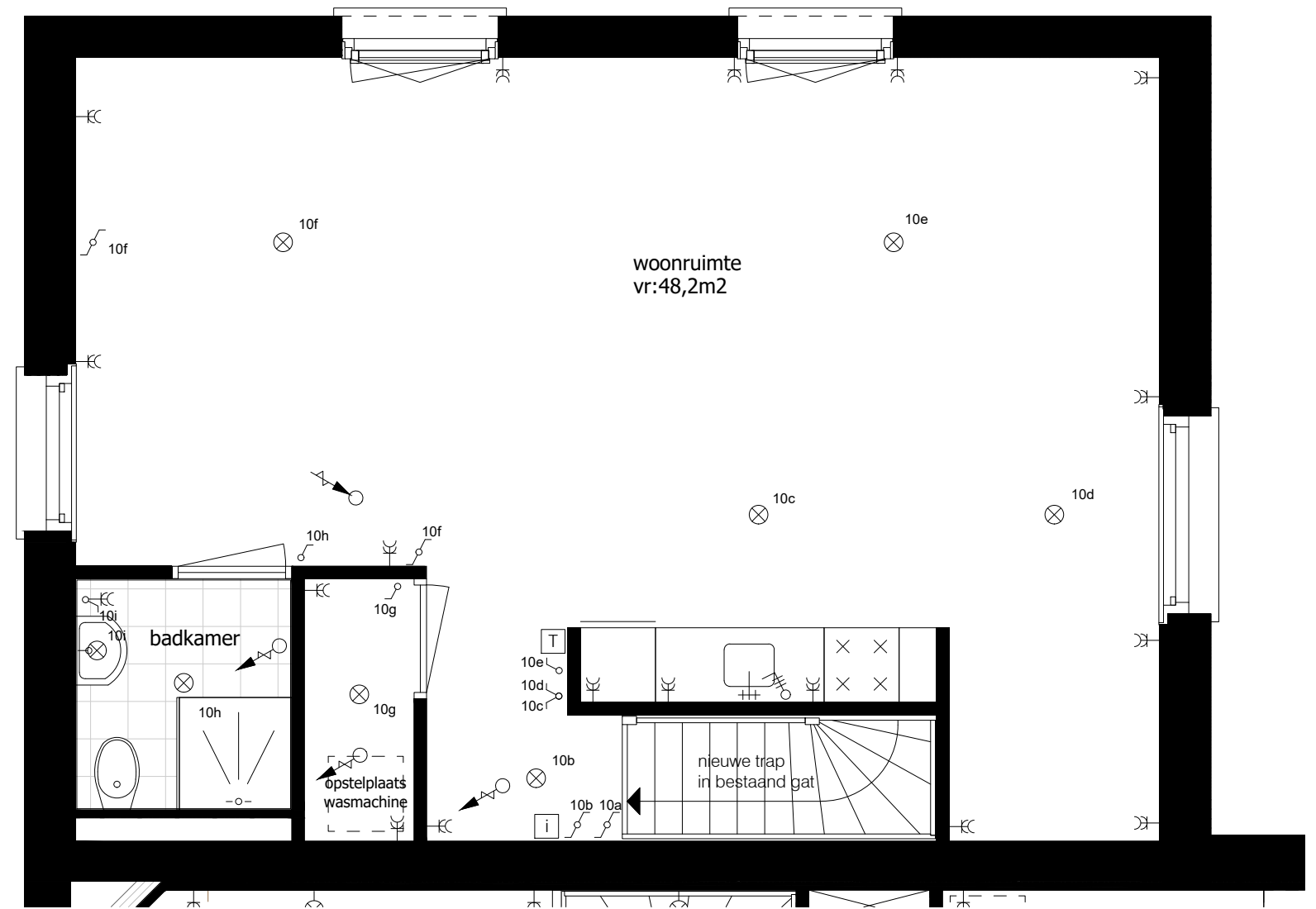
2e verdieping 1:50
