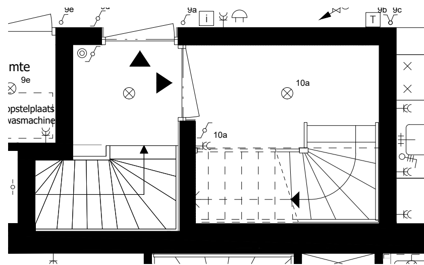
Entree (1e verdieping) 1:50
